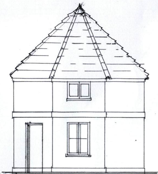
NE ELEVATION 1:100
